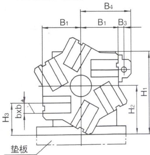
A 向 JLD6-C0625~C6125
