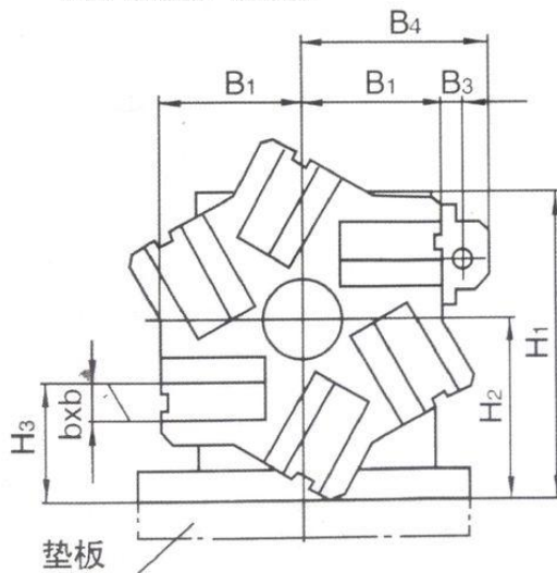
A 向 JLD6-C0625~C6125
