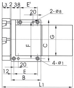
A 向 JLD6-C0625~C6125
