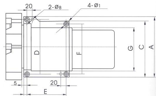
A 向 JLD6-C6132~C6150
