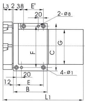
A 向 JLD6-C0625~C6125
