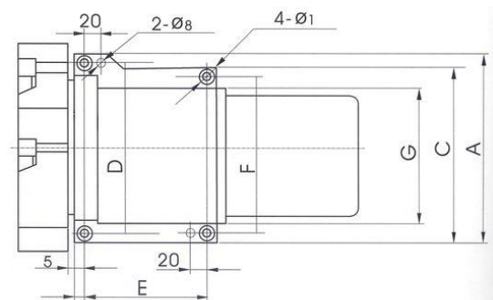
A 向 JLD6-C6132~C6150
